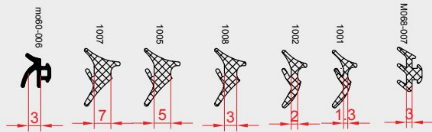
اندازه‌ی شیشه و لاستیک‌ها Gaskets and Glass Dimension
