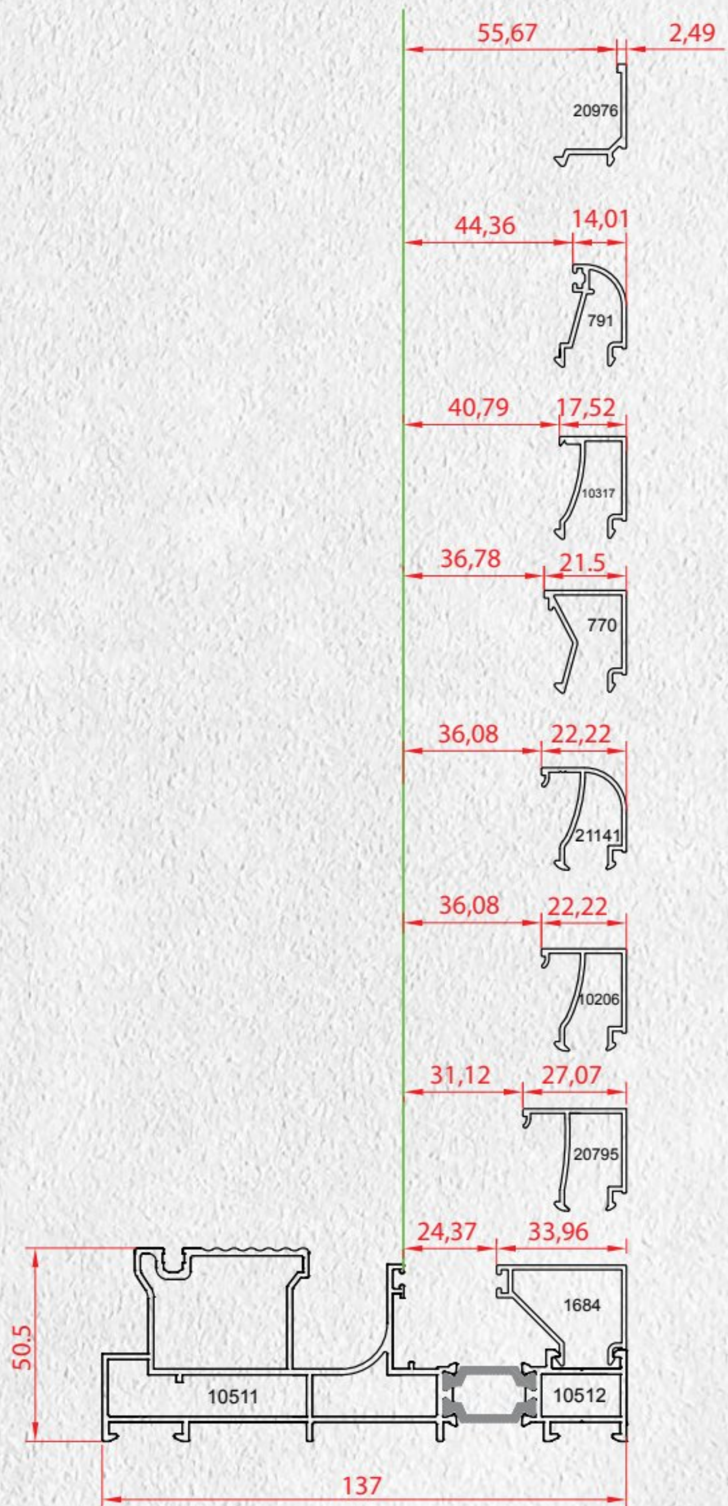
اندازه‌ی شیشه و لاستیک‌ها Gaskets and Glass Dimension
